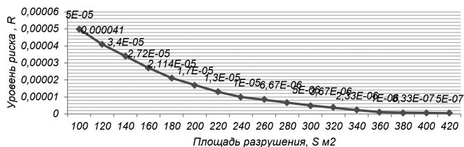
Рис.1. Зависимость уровня риска от площади разрушения
