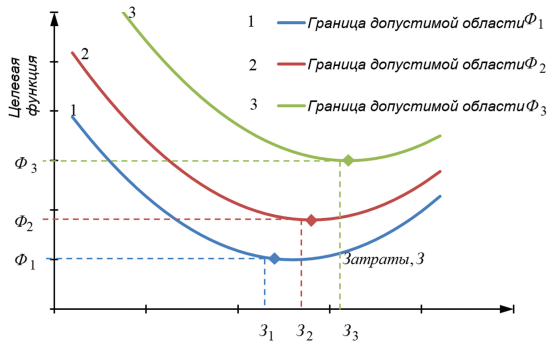
Рис. 2. Области оптимальных решений плиты в зависимости от вида целевой функции
