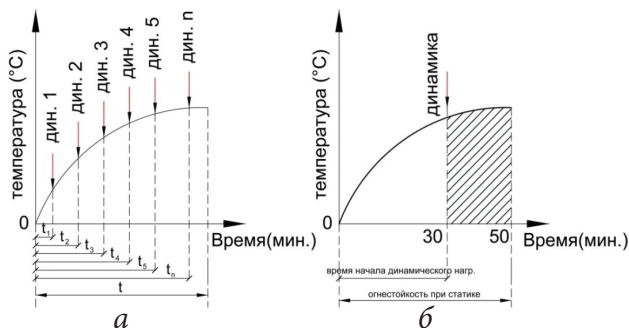
Рис. 5. Варианты динамического нагружения элементов при пожаре: а — схематичное приложение динамической нагрузки; б — огнестойкость колонны при разных типах нагружений
