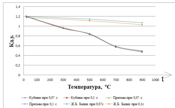
Рис. 3. График зависимости коэффициента динамического упрочнения бетонных кубиков, призм и железобетонных балок от огневых воздействий
