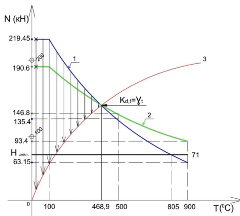
Рис. 4. График прочности железобетонной колонны при стандартном температурном режиме: 1 — динамической; 2 — статической; 3 — кривая температуры пожара по ISO 834
